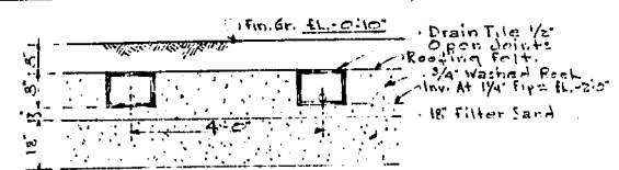
DRAIN BED DETAIL N.T.S.
