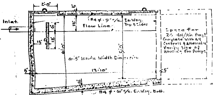
SEPTIC TANK SECTION Scale: N.T.S.
